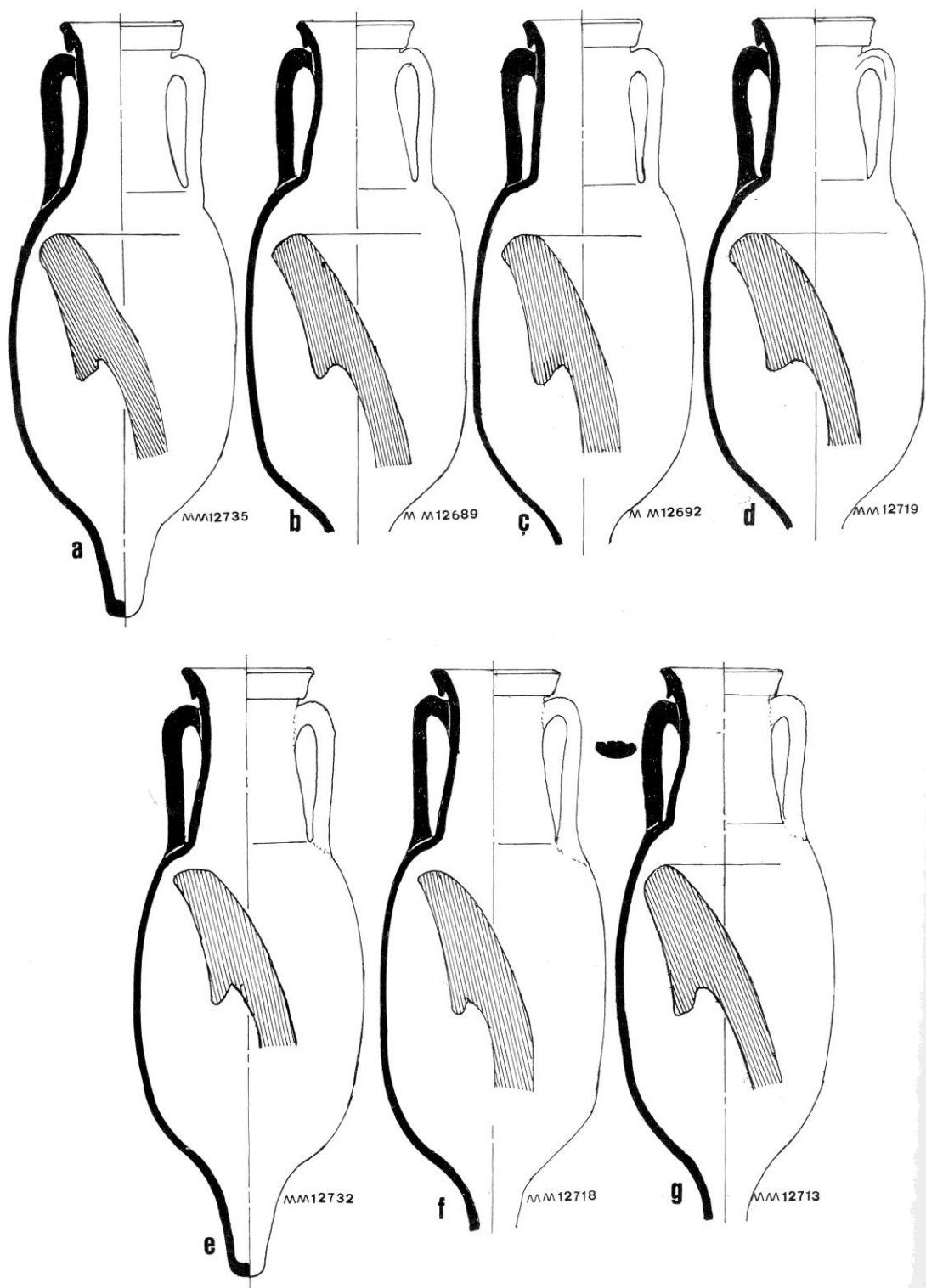
ig. 22.- GRUP "B": Set àmfors Dressel 7, variant de l'orla Oberaden, 3, del Cabrera 5
