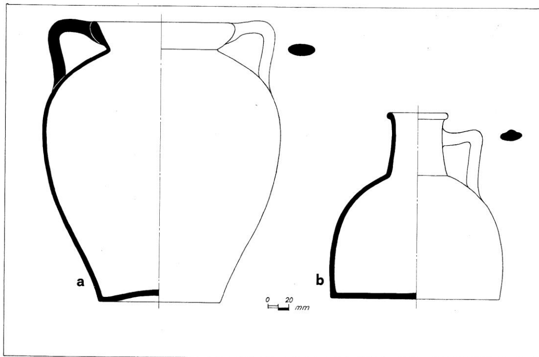
Figura 15. Peces de ceràmica comuna del Moro Boti
