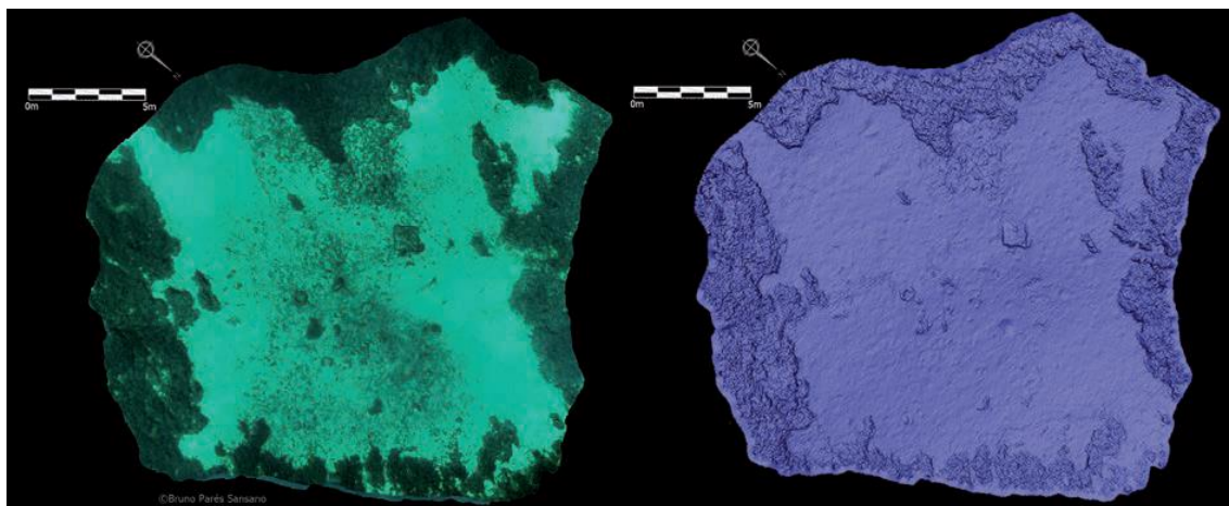
Ortofotografía y modelo tridimensional del Cabrera III (Riera et al, 2016)
