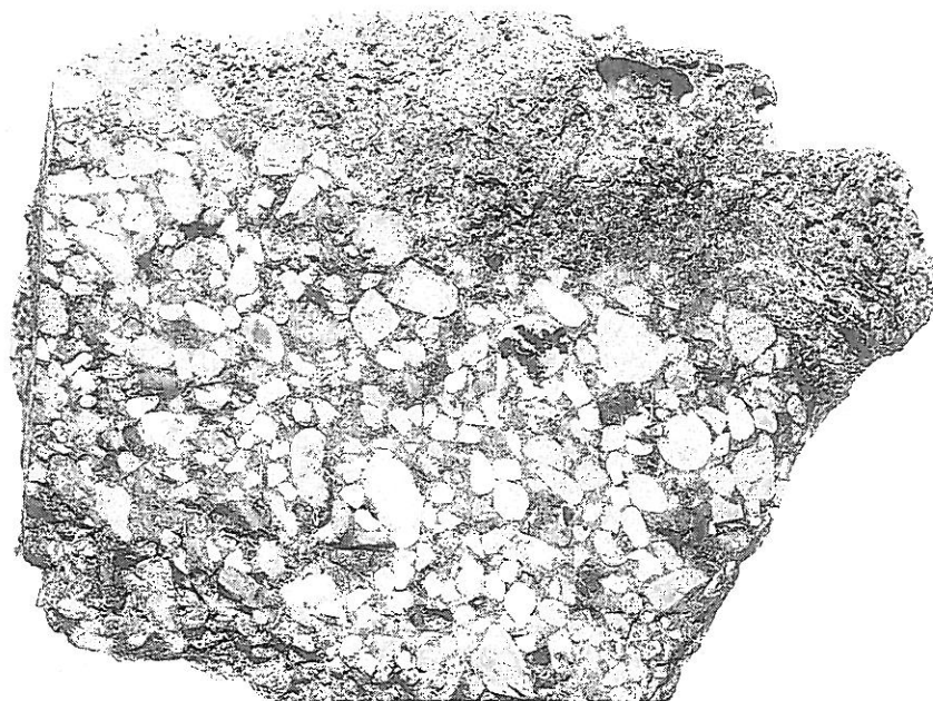
1. - OUVRAGE AQT. BOUÉE Q. — BLOCS DE LA JETÉE. (Prélèvement N° 14. Grandeur naturelle). Poudingue à base de petits galets de silex et croûte de calcaire concrétionné dépourvu de galets.
