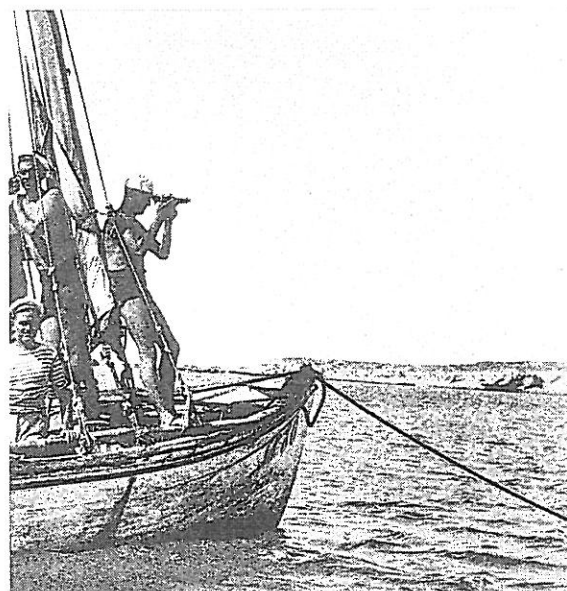
4. - Cercle hydrographique. Officier de marine (Ens. Guès) situant les points étudiés par le scaphandrier.
