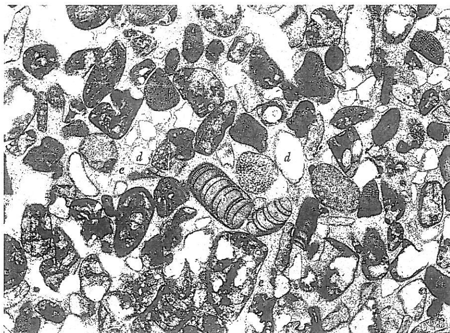
2. - ROCHE DE L'ILE DE TYR. (Prélèvement N° 40. Section mince agrandie 25 fois). a , Fragment calcaire remanié et arrondi ; b , Amphiroa ; c , Foraminifère ; d , Quartz ; e , Gangue de calcite micro-grenue.
