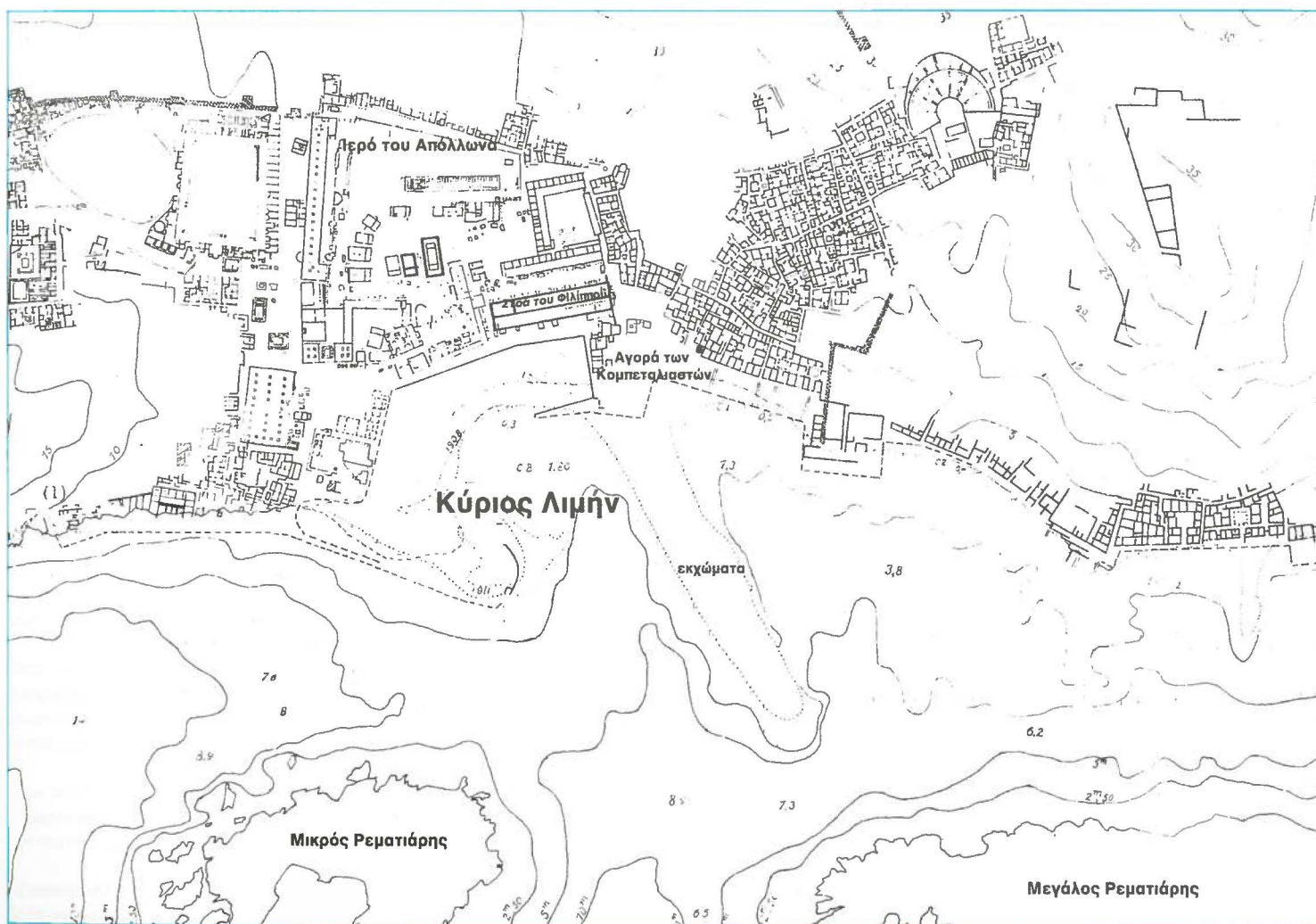
Εκ. 2. Κάτοψη της περιοχής του κεντρικού λιμένα (σχέδ. Γ. Πάντζαρη).
