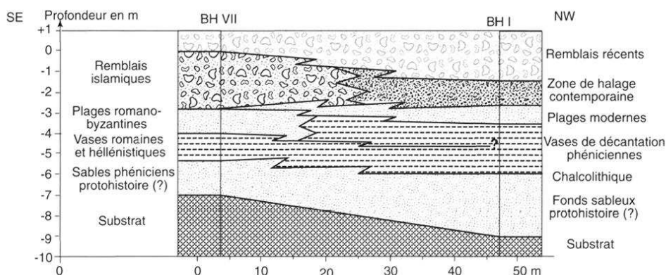
FIG. 6 - PROFIL SIMPLIFIÉ BH VII - BH I
