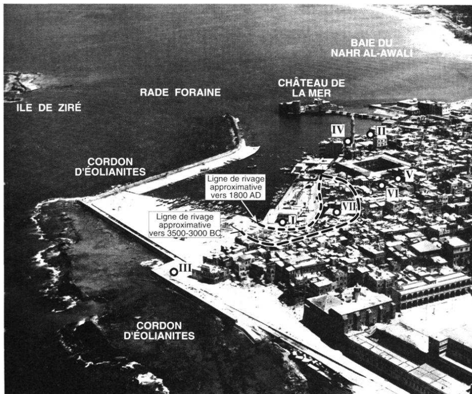
FIG. 7 - ÉVOLUTION PROBABLE DE LA LIGNE DE RIVAGE DEPUIS 5000 ANS. ÉTUDE PALÉOENVIRONNEMENTALE DU PORT ANTIQUE DE SIDON. PREMIERS RÉSULTATS DU PROGRAMME CEDRE
