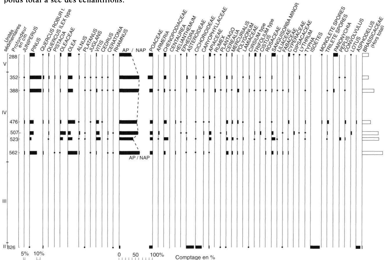
FIG. 4 - DIAGRAMME POLLINIQUE DE LA CAROTTE BH I (AP = pollen arboréen et NAP = pollen non arboréen)
