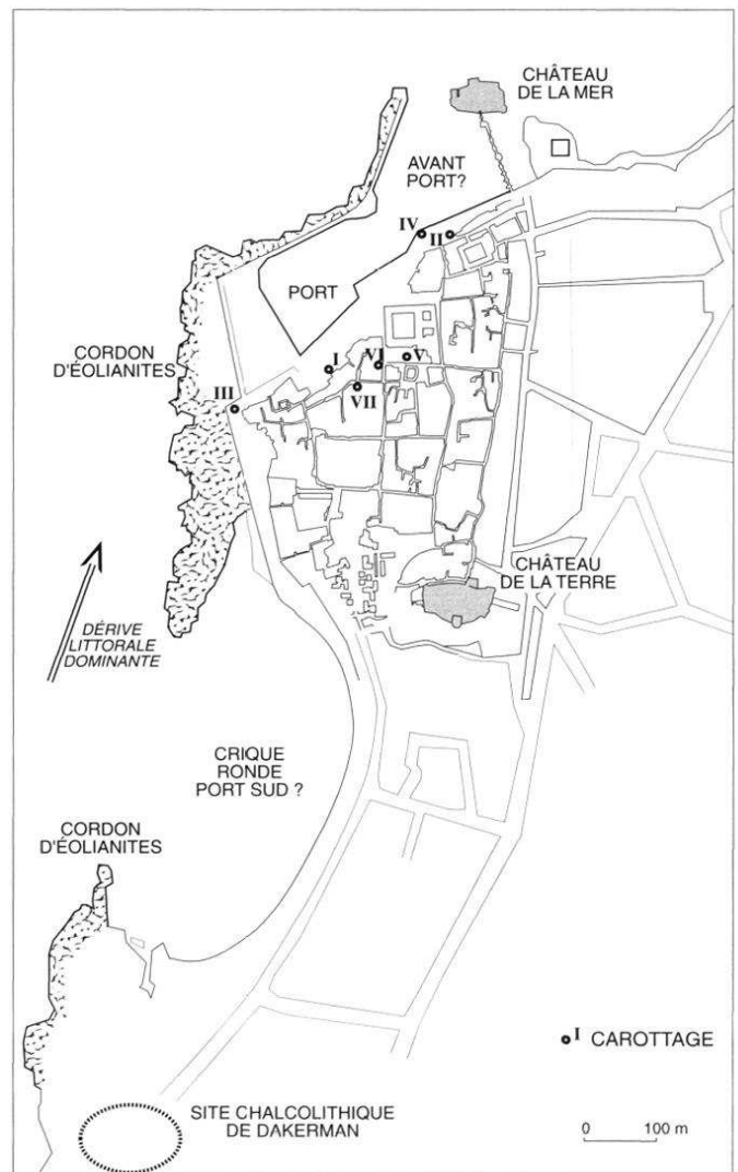
FIG. 2 - LOCALISATION DES CAROTTAGES DANS LE PORT ANTIQUE DE SIDON
