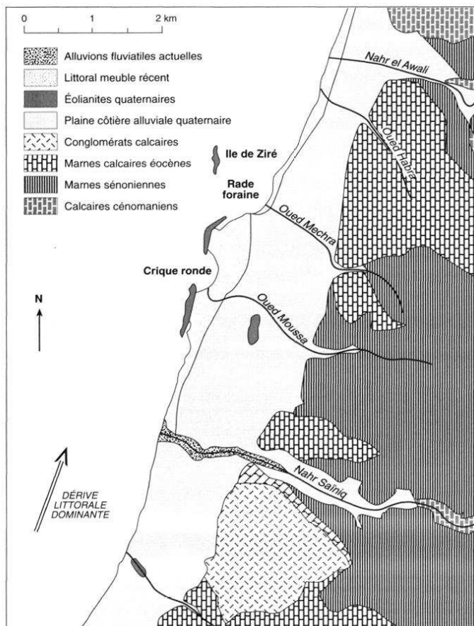
FIG. 1 - CARTE GÉOLOGIQUE SIMPLIFIÉE DE LA RÉGION DE SAÏDA (d'après DUBERTRET, 1949)
