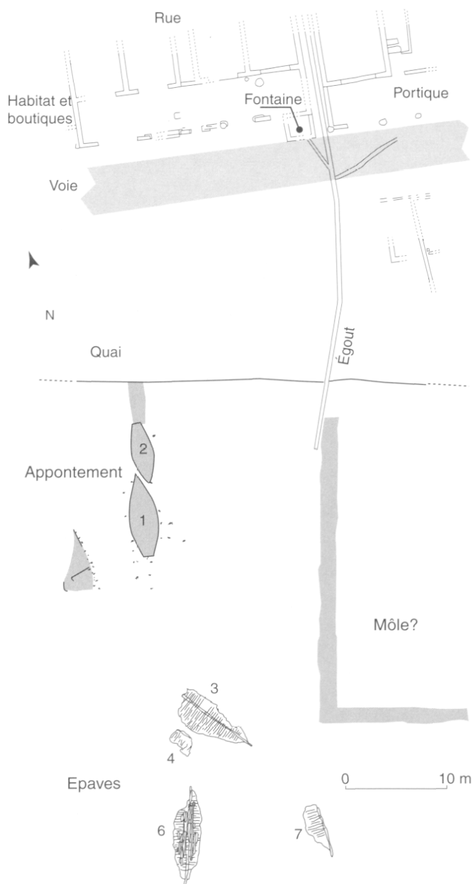
FIG. 4 - PLAN DES AMÉNAGEMENTS PORTUAIRES D'ÉPOQUE ROMAINE DÉCOUVERTS À TOULON. (d'après Gallia informations , 1990, p.240)
