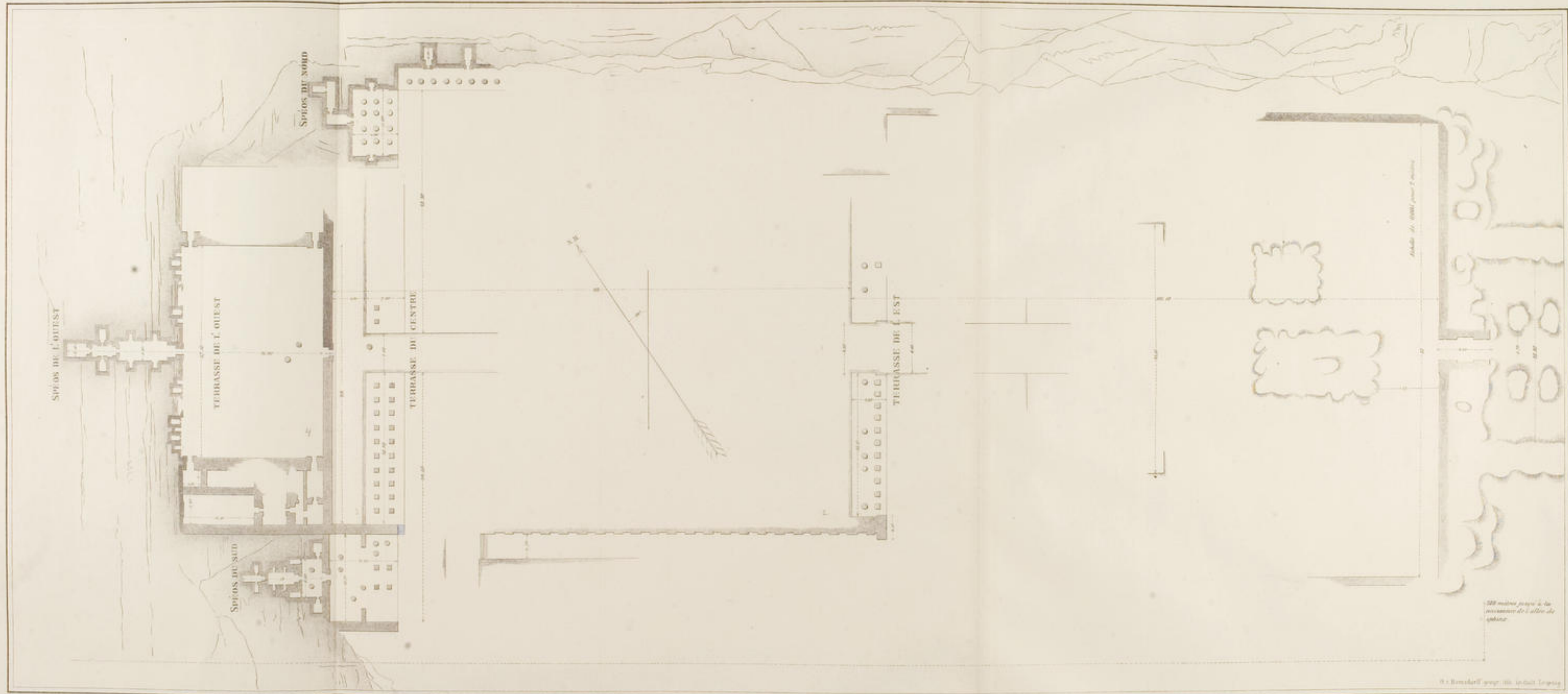
ÉTAT DES LIEUX APRÈS LES FOUILLES DE 1858.
