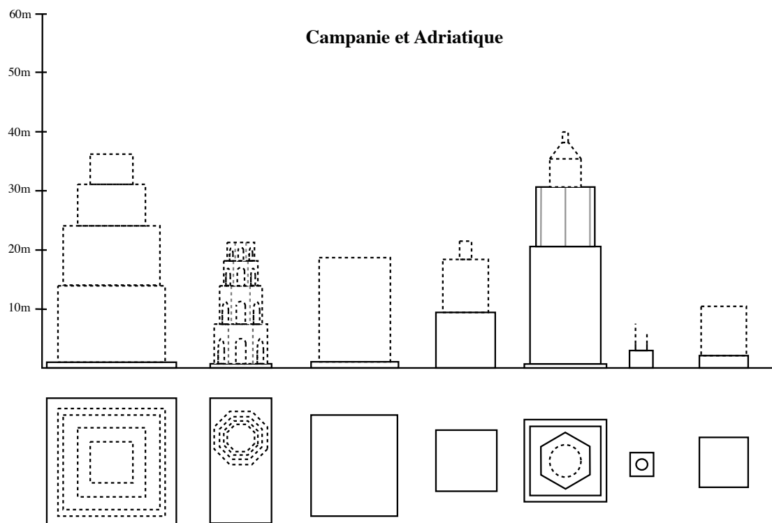
1. Phare de Claude, Portus; 2. Phare de Trajan, Portus; 3. Tor Boacciana, Ostia; 4. Misene; 5. Capri, Punta della Campanella; 6. San Felice Canale
