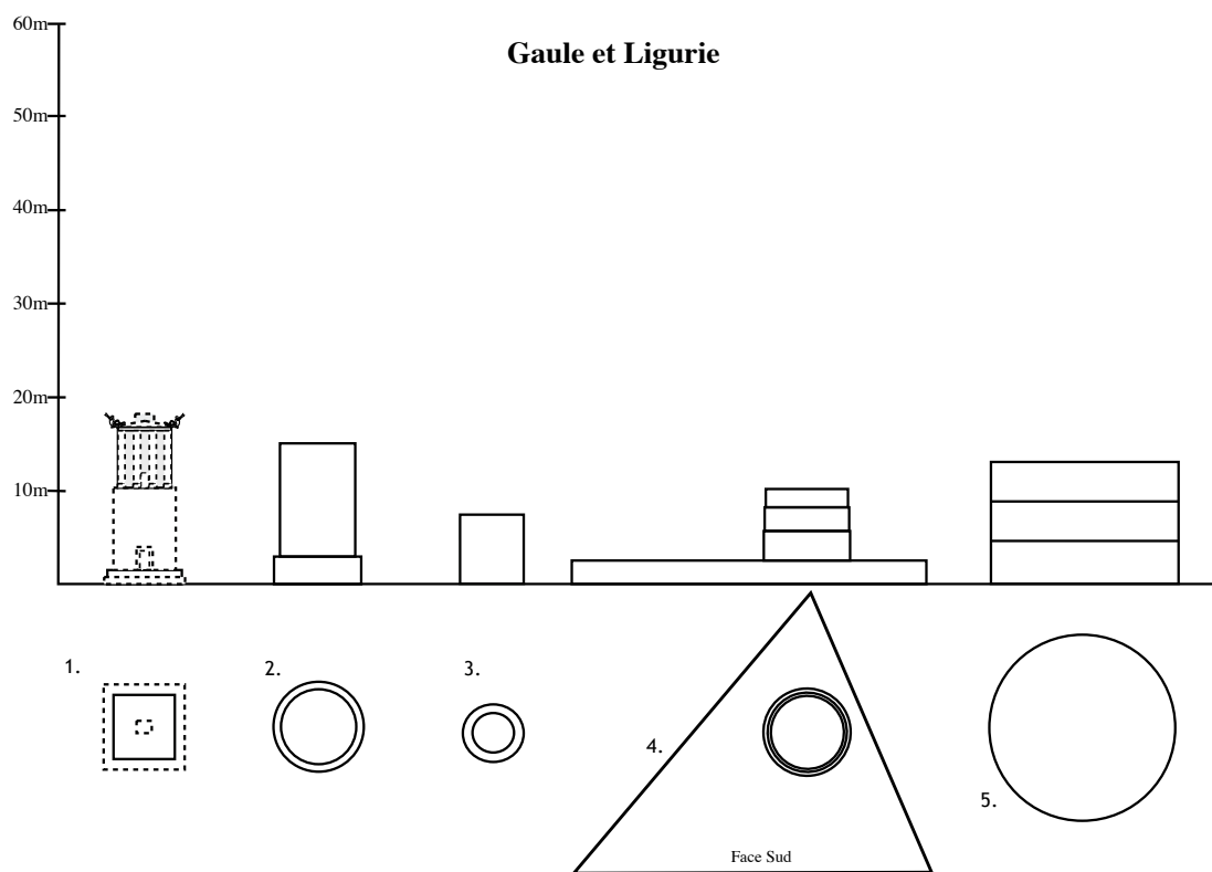
1. Monument aux Tritons, Fréjus; 2. phare du Lion de Mer; 3. Tour St anne, île Ste Marguerite; 4. phare de l'île de Bergeggi; 5. Phare de Trajan, Centumcellae
