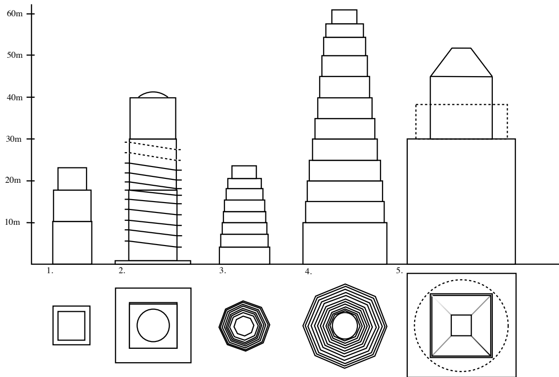
1. Torre Augusto, Gjon; 2. Torre Hercules, La Corogne; 3. Phare de Douvres; 4. Turris Ordens, Boulogne-sur-mer; 5. Phare de Gadès
