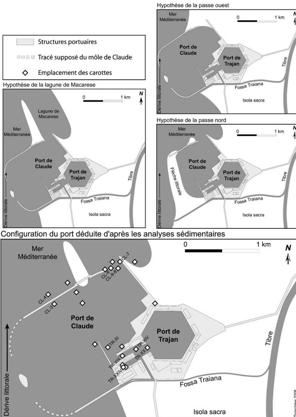
Portus- Hypothèses sur la configuration du port de Claude et résultats basés sur les analyses sédimentaires. Extrait J.P. Goiran et H. Tronchère MEFRA – 120/1 – 2008, p. 269. fig 29
