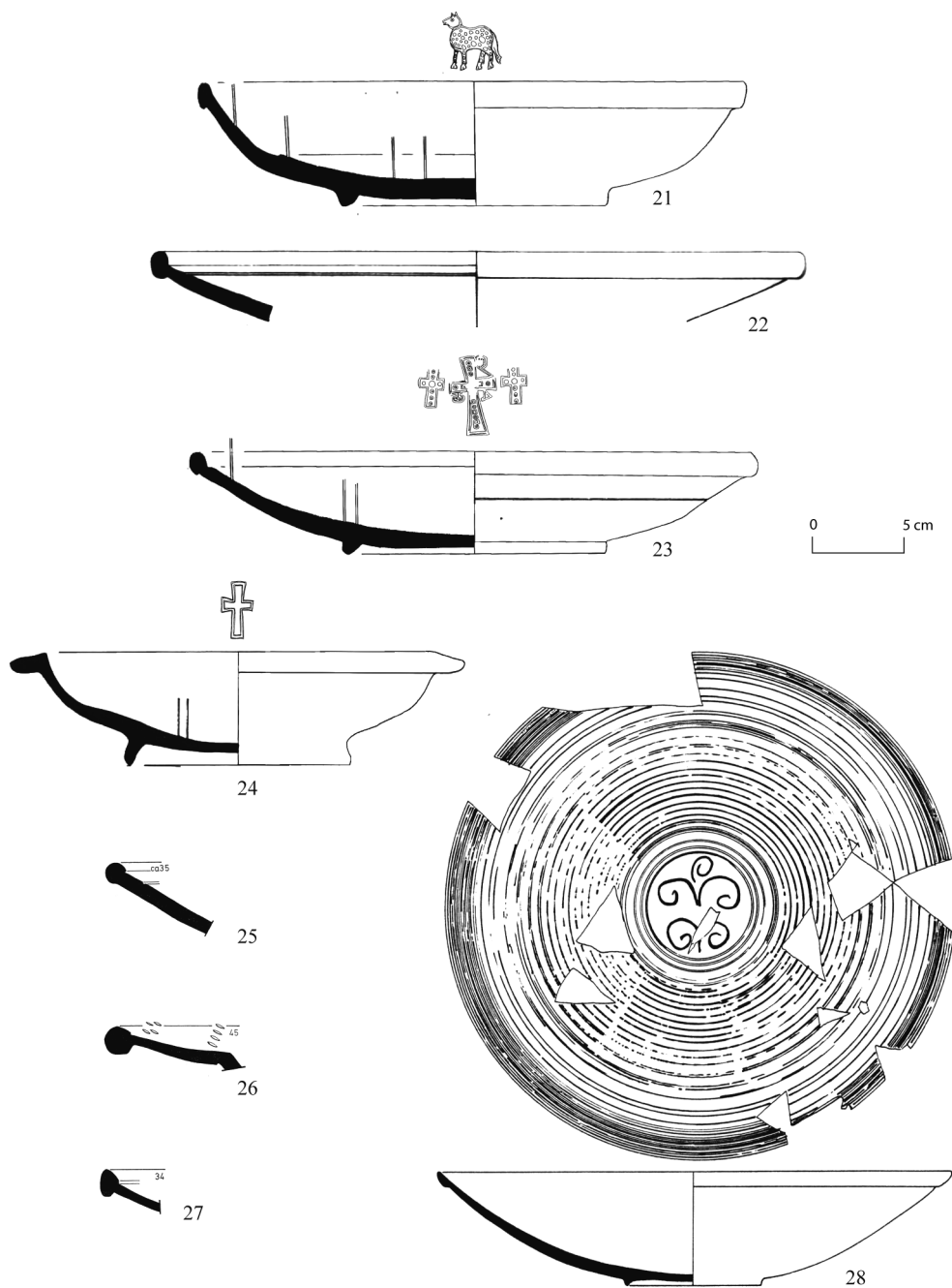
Fig. 3. Sigillées africaines importées en Égypte.
