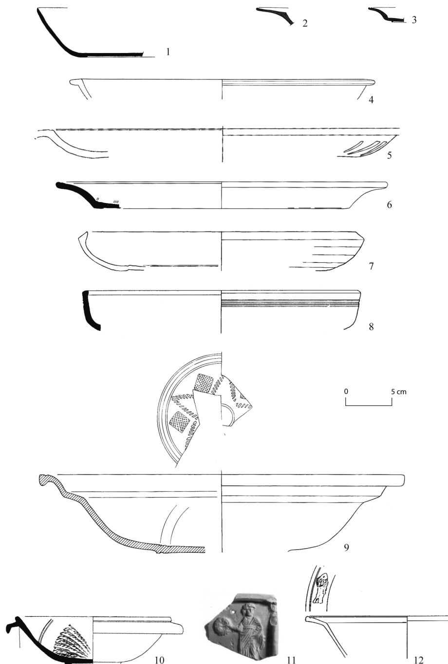
Fig. 1. Sigillées africaines importées en Égypte.
