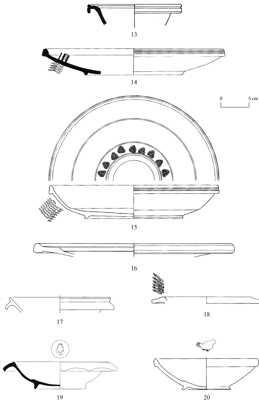
Fig. 2. Sigillées africaines importées en Égypte.
