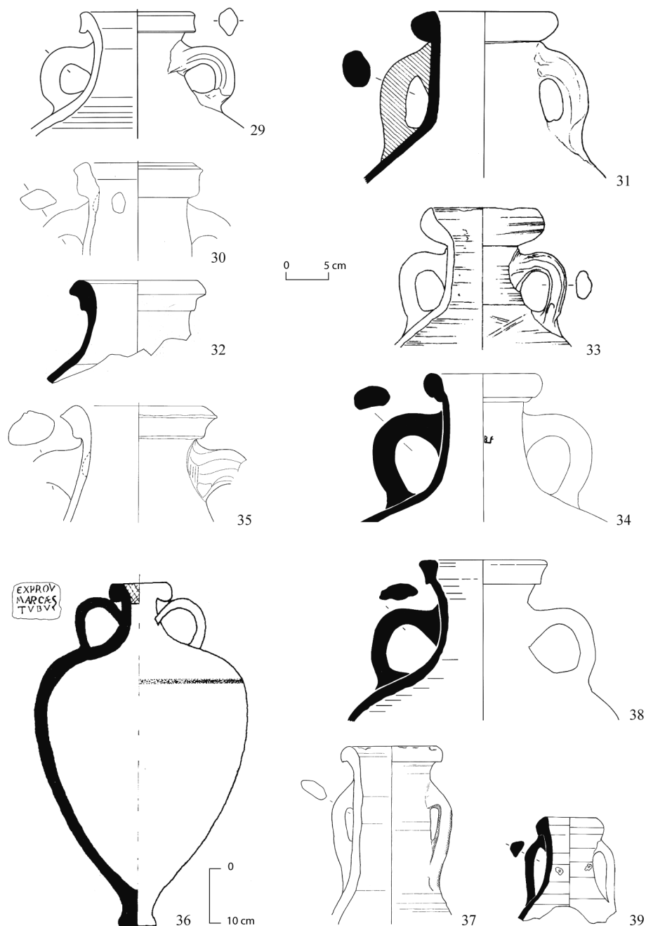
Fig. 4. Amphores africaines importées en Égypte.
